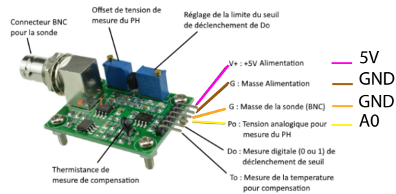
carte Logo_PHsensor V1.1
